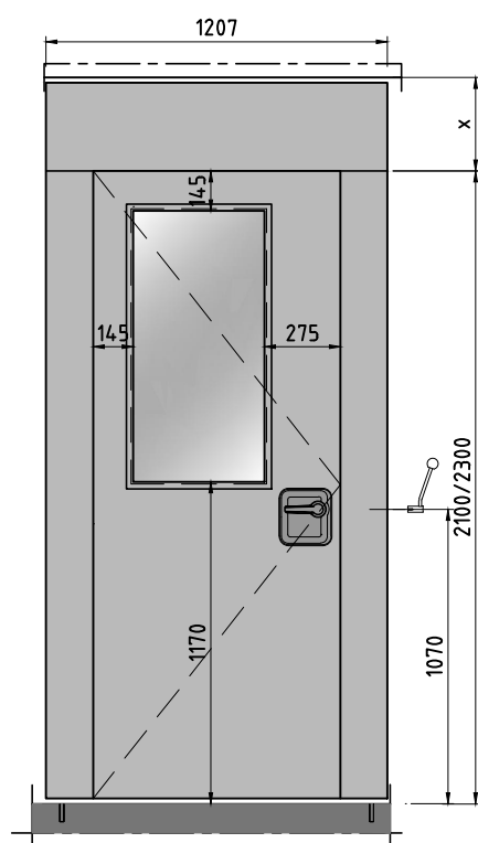
Deurpaneel met standaard glasopening
