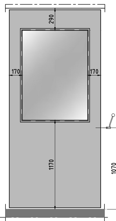
Basispaneel met standaard glasopening
