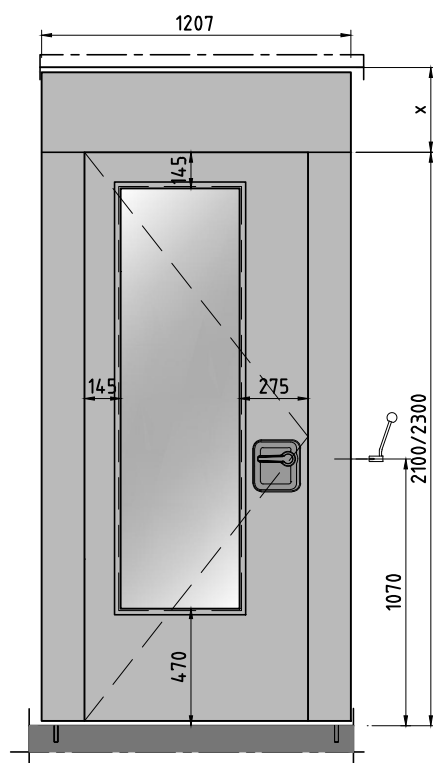
Deurpaneel met maximale glasopening
